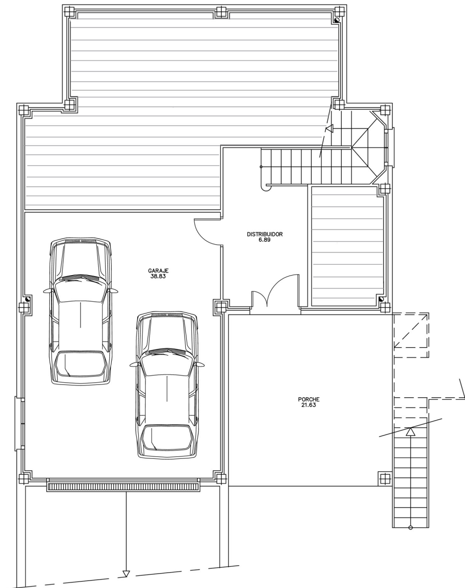
PLANTA SÓTANO
